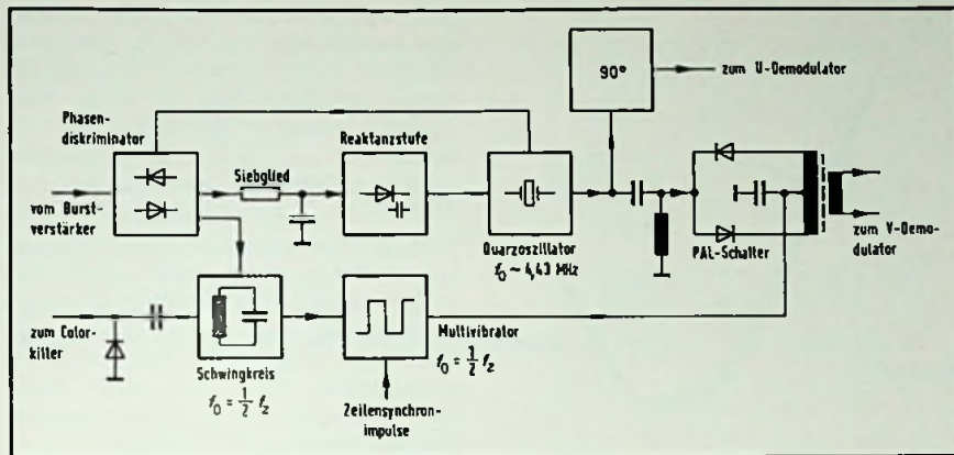
Bild 18. Blockschialtung der Referenzträgererzeugung und Phasenumschaltung (Grundlg)
