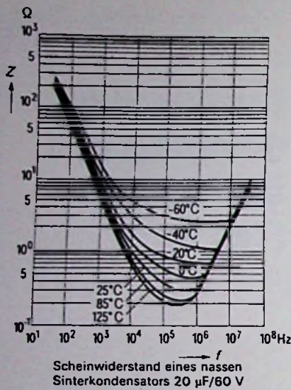
Bild 1.66. Scheinwiderstand eines nassen Tantalelkos (links) und eines trockenen Tantalelkos (rechts) in Abhängigkeit von der Frequenz (Siemens)
