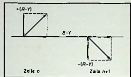
Bild 11. So werden die R - Y -Komponenten zellenweise umgeschaltet (Verfasser)
