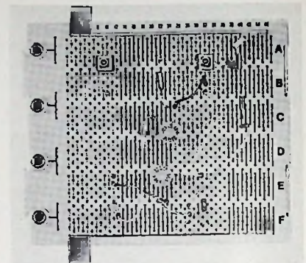
Experimentierplatte XP 101 von Hirschmann mit aufgebauter astabiler Kippstufe
