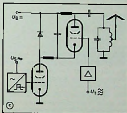
Bild 1. Amplitudenmodulationsverfahren bei Hochleistungssendern: a) mit Gegentakt-B-Modulationsverstärker b) durch Doherty-Modulation c) mit PDM-Verstärker
