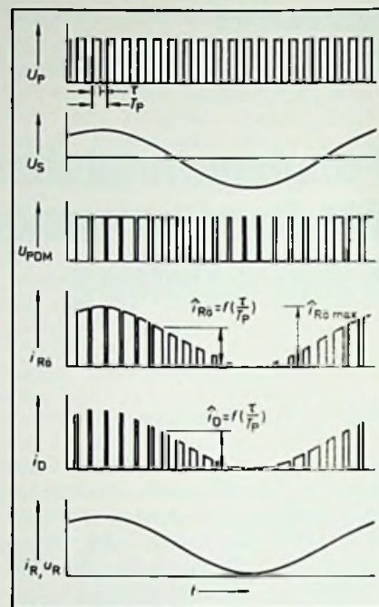
Bild 4. Signalverlauf beim PDM-Verstärker
