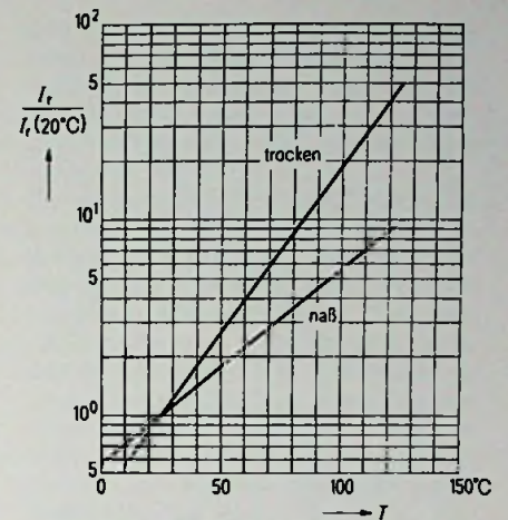
Bild 1.69. Temperaturabhängigkeit des Reststromes beim Tantalelko; nasser und trockener Typ (Siemens)
