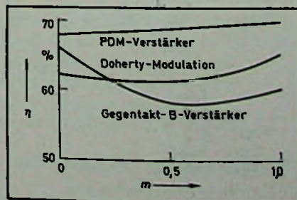
Bild 2. Gesamtwirkungsgrad bei amplitudenmodulierten Hochleistungssendern
