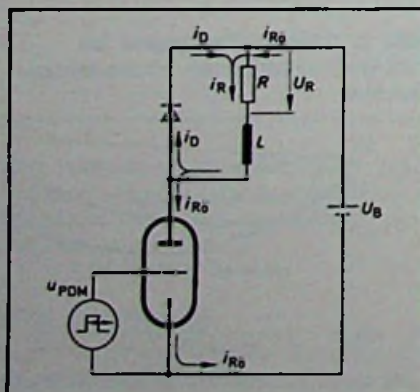
Bild 3. Grundschialtung des PDM-Verstärkers
