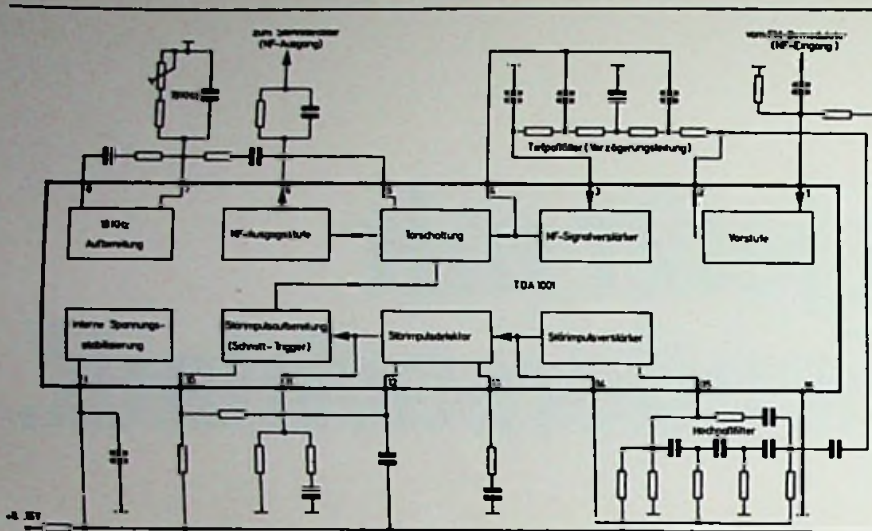
Bild 7. Blockschema der EIC-Schaltung von Becker
