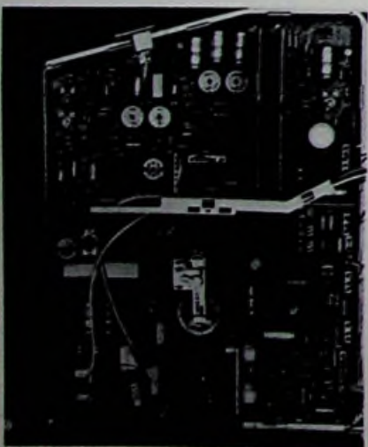
Bild 6. Großsignalplatine des Philips-farbfernseh-Chassis K 9/i
