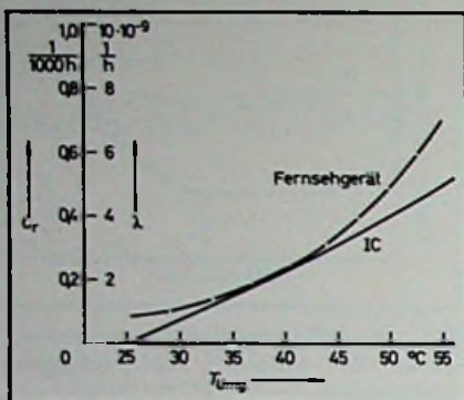
Bild 4. Ausfallrate in Abhängigkeit von der Umgebungstemperatur
