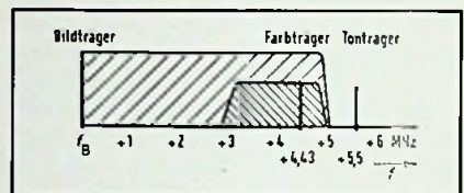
Bild 12. Stellung des Farbhilfsträgers innerhalb des Videobandes (Grundig)
