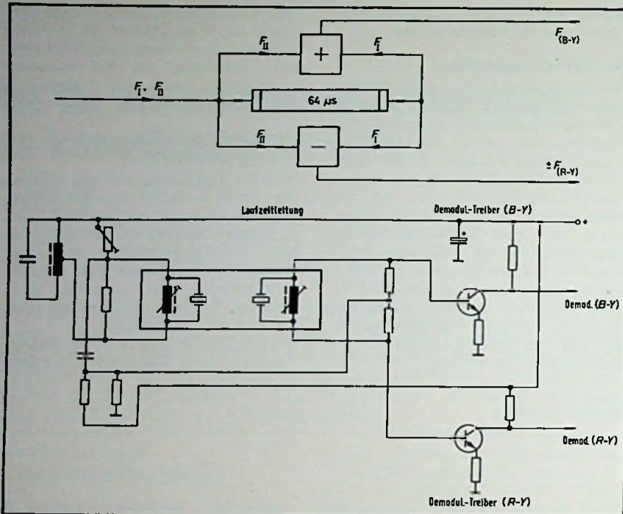
Bild 16. Prinzip und Schaltungsausschnitt des Pal-Demodulators. F_i stellt das verzögerte, F_{ii} das unverzögerte Signal dar (Verfasser)
