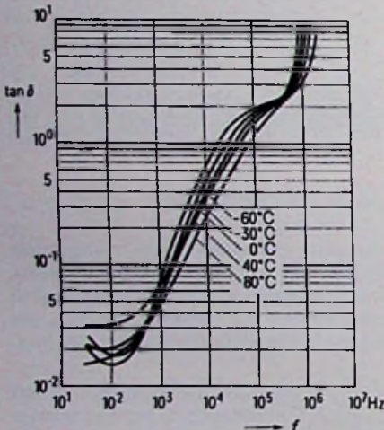
Bild 1.67. Verlustfaktor \tan \delta eines trockenen Tantalelkos in Abhängigkeit von der Frequenz (Siemens)
