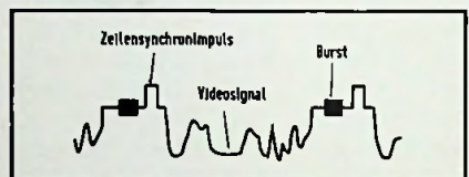
Bild 13. Zeilensynchronimpuls mit Burst (Schaub-Lorenz)
