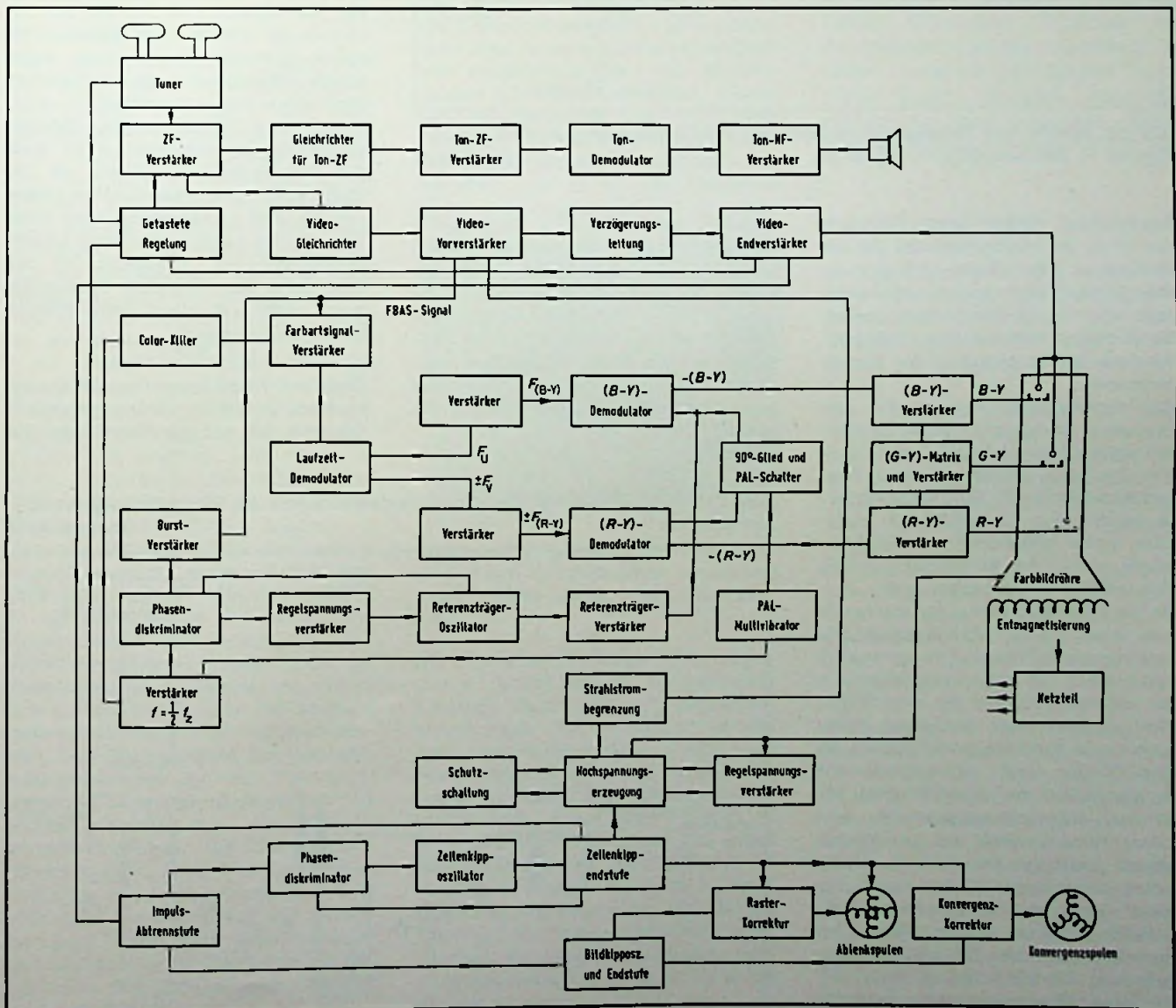
Bild 15. Blockschaftbild eines Farbfernsehempfängers (Grundrig)
